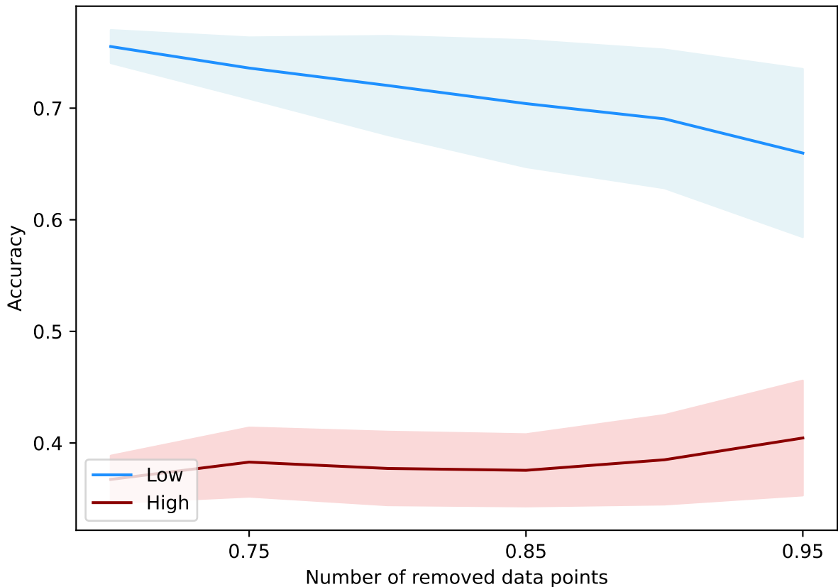
DataAttrOpt(10000, 0.03, 15, inf, +b, alpha=1.0) - imdb-embeddings
